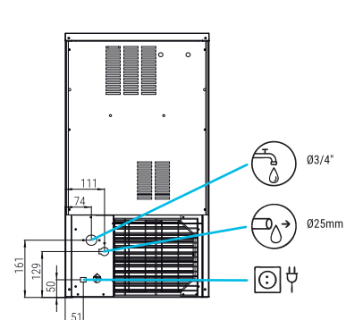
ΠΙΣΩ ΟΨΗ
